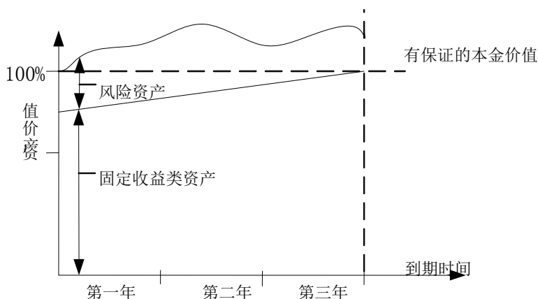
图 1 CPPI 策略下的本金保障
